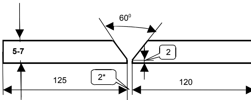
Fig.1. Secțiunea îmbinării cap la cap.
