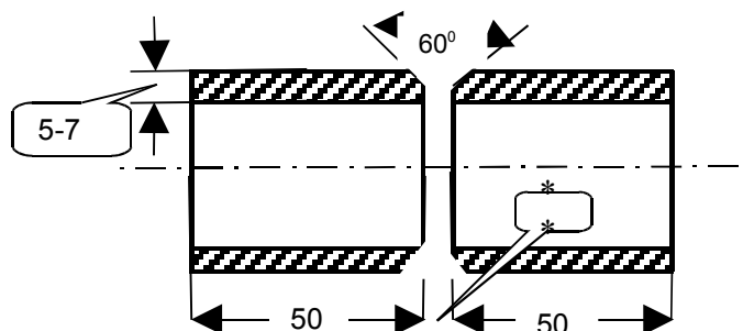
Figura 2. Forma îmbinării cap la cap pentru procedeul WIG
